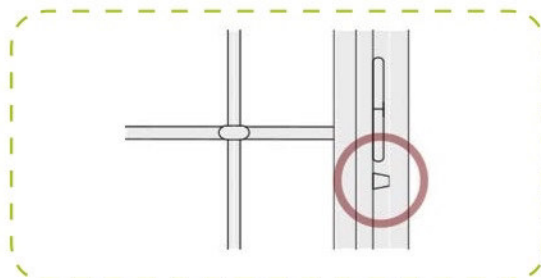
1. Perni antistrappo
