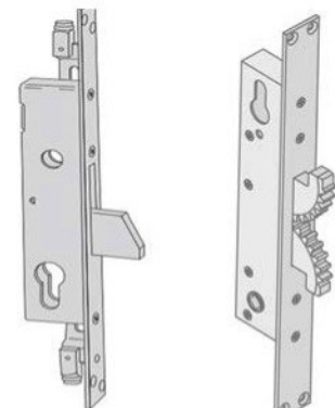
Dettaglio serratura cilindro europeo
