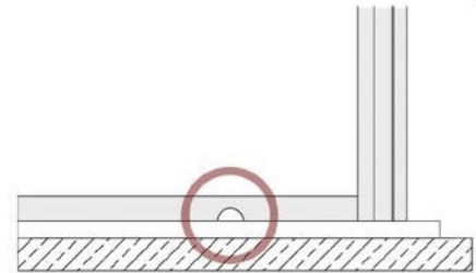
2. Sezione circolare per il deflusso dell'acqua piovana
